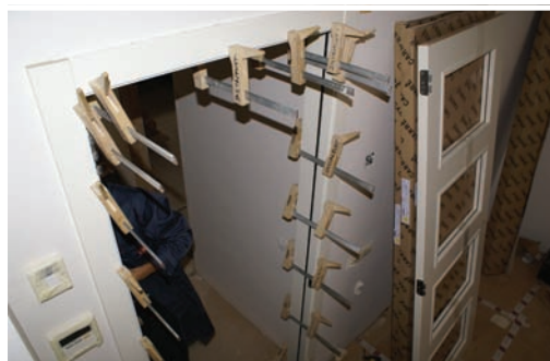
Fijar definitivamente. Definite fixation. Fixation définitive.
