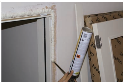
Sellar el hueco con espuma poliuretano. Seal the gaps with polyurethane foam. Sceller avec mousse de polyuréthane.
